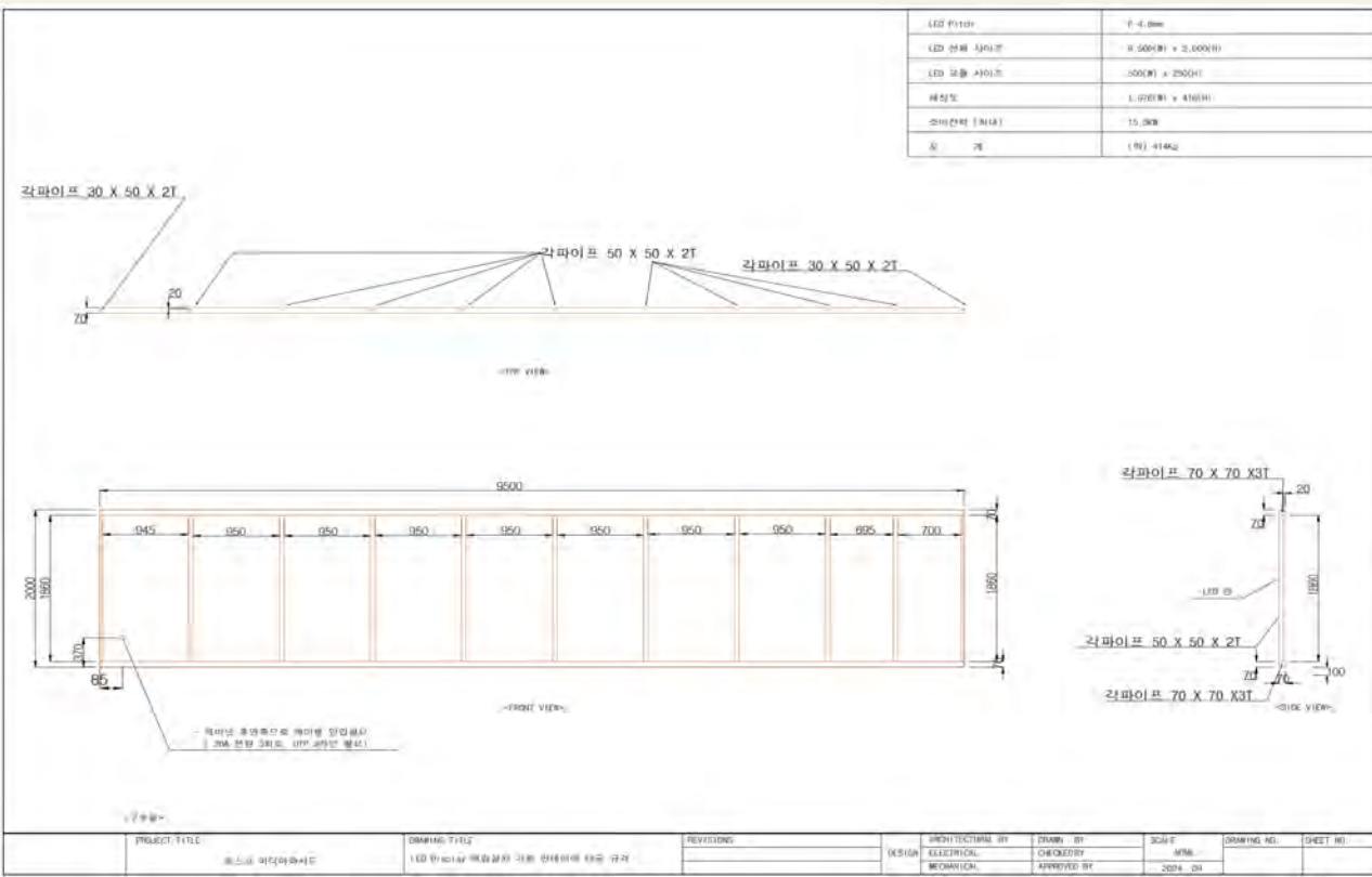
보강 도면 작업
